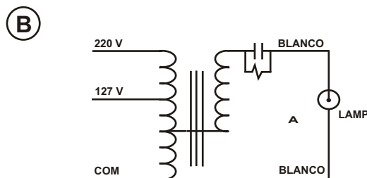
DIAGRAMAS: CIRCUITO ADELANTADO
