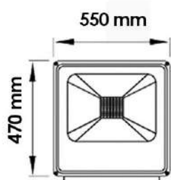
ALZADO FRONTAL
