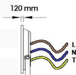
ALZADO LATERAL
